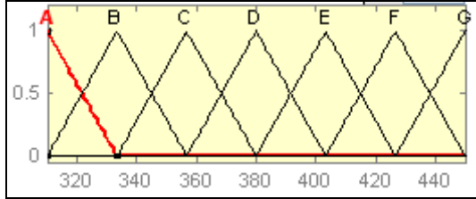
Şekil 4. Çimento dozajına ait üyelik fonksiyonları (kg)
