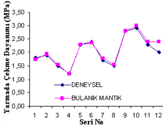
Şekil 8. Çimento dozajının yarmada çekme dayanımına etkisi
