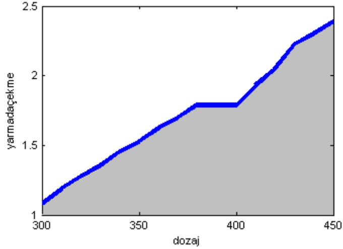
Şekil 8. Çimento dozajının yarmada çekme dayanımına etkisi
