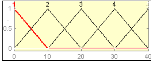
Şekil 5. Uçucu kül ikame miktarına ait üyelik fonksiyonları
